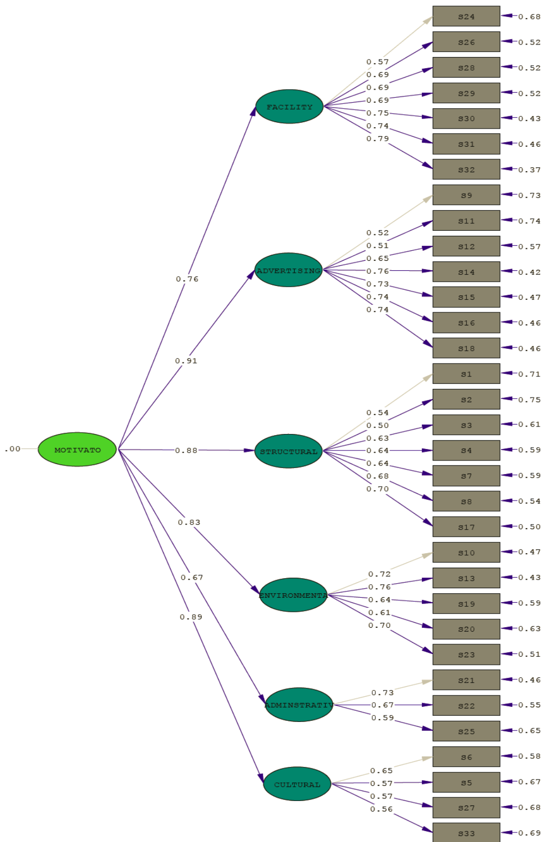
شکل ۲. نتایج تحلیل عاملی تأییدی مرتبه دوم با بار عاملیها
