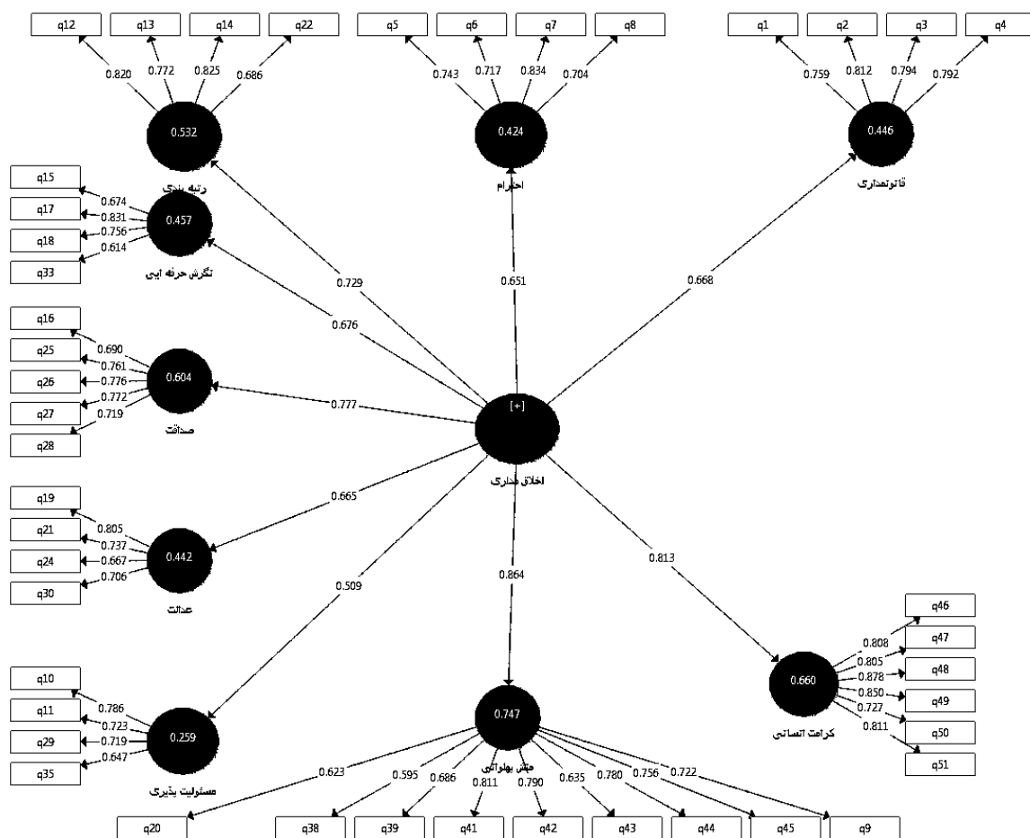
شکل ۲. مدل مفهومی در حالت تخمین بارهای عاملی
